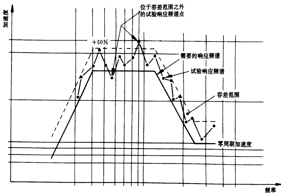
图2 所需响应谱的典型对数曲线
